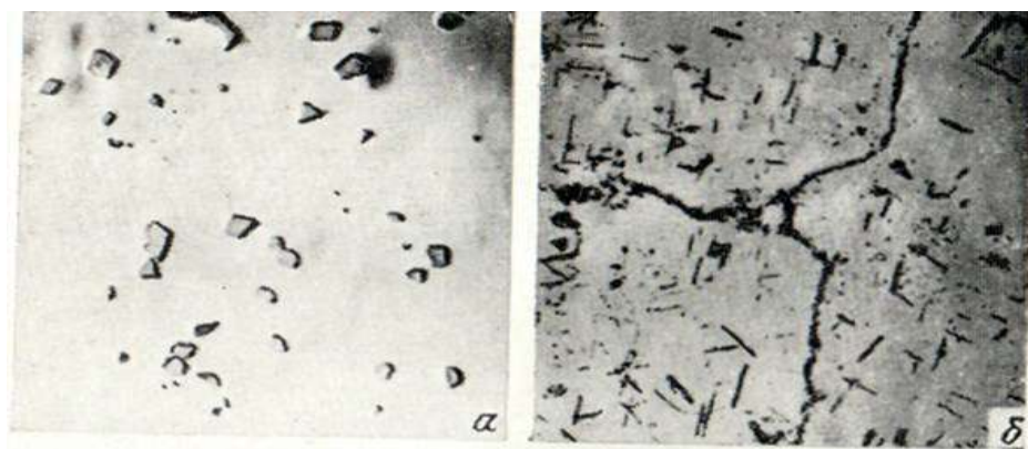
Рисунок 2. Вид карбидных фаз в зависимости от соотношения Al и Ti в сплаве, \times 500 : а – 4,5 % Al, 3% Ti; б – 7 % Al, 3% Ti
