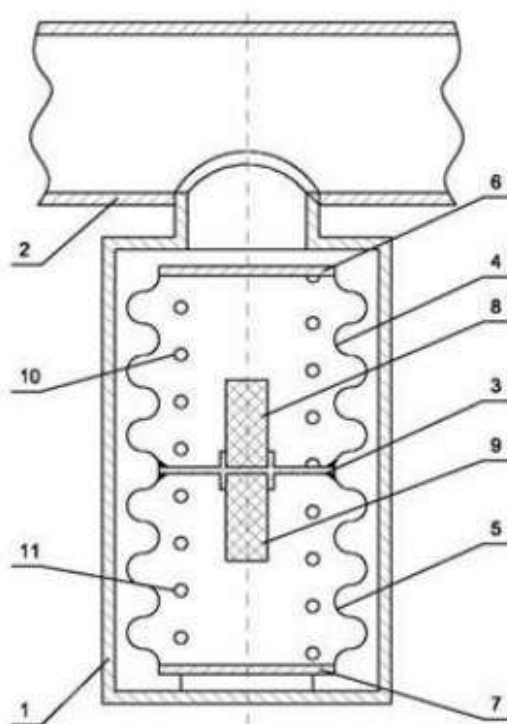
Рисунок 3. Сильфонный демпфер
