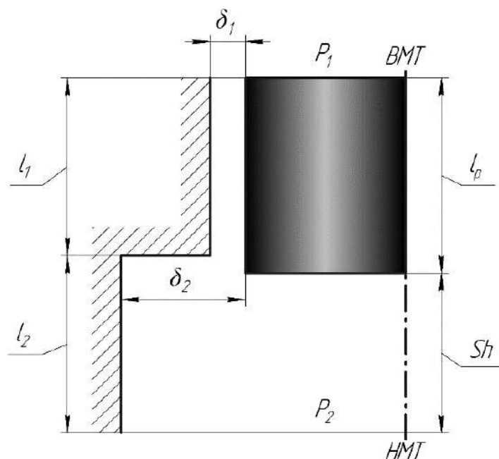
Рисунок 3. Ступенчатое щелевое уплотнение
