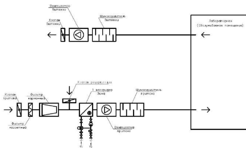
Рисунок 3. Принципиальная схема лабораторного стенда для выполнения экспериментальных исследований аэродинамических характеристик отдельных элементов системы воздуховодов
