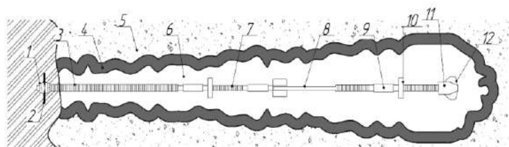
Рисунок 1. Схема закрепления микро-свай из ТВШ в грунте: 1-фиксирующая гайка; 2-опорная плита; 3-защитная трубка из ПВХ; 4-зона первичной инъекции грунта; 5-вмещающий грунт; 6-цементное тело; 7-ребристая штанга; 8-внутренний канал штанги; 9-соединительная муфта; 10-распорка; 11-буровая коронка; 12-инъекционное отверстие;
