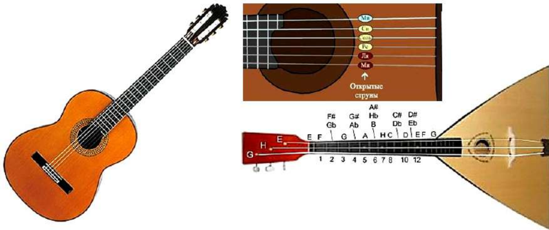
Рисунок 1. Классическая испанская гитара (строй гитары e, h, g, d, a, e) и расположение нот по ладам балалайки (строй e, h, g)
