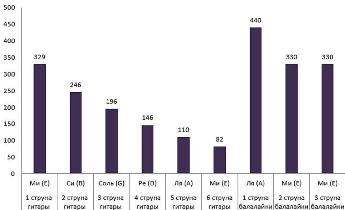
Рисунок 7. Диаграмма частот колебаний струн гитары и балалайки
