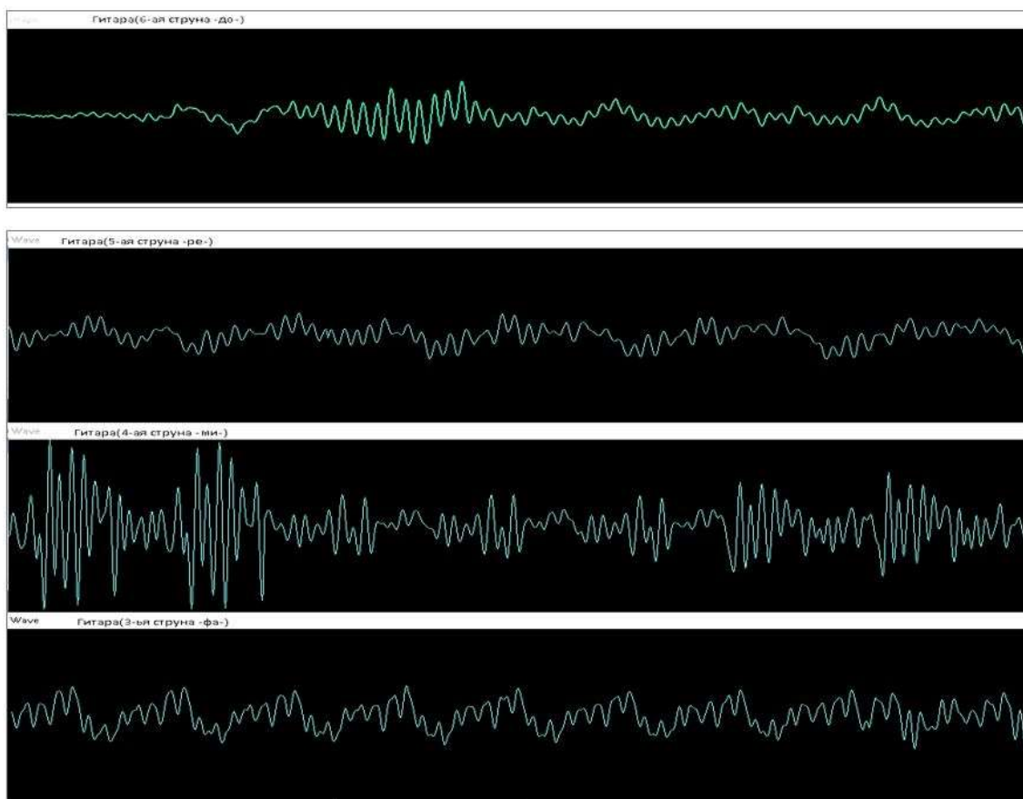
Рисунок 9. Осциллограммы колебаний 3-6 струн гитары зафиксированные электронным осциллографом Frequency Analyzer
