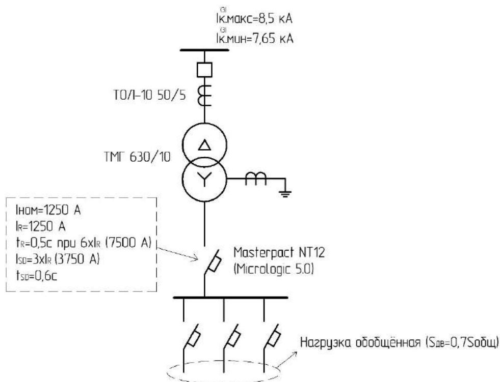
Рисунок 2. Исходные данные к расчёту релейной защиты трансформатора
