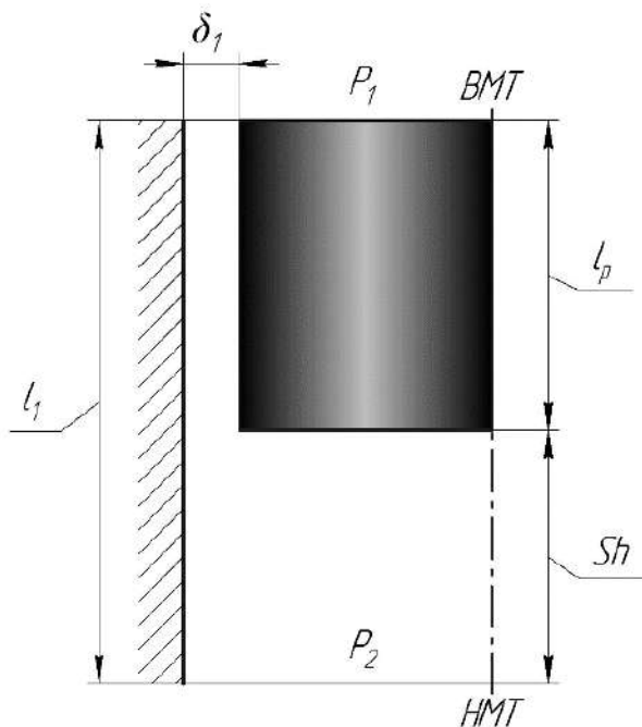
Рисунок 1. Гладкое концентричное щелевое уплотнение
