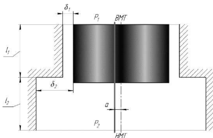
Рисунок 4. Эксцентричное расположение щелевого уплотнения ступенчатого вида
