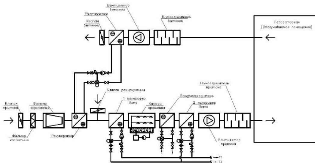
Рисунок 2. Принципиальная схема приточно-вытяжной установки
