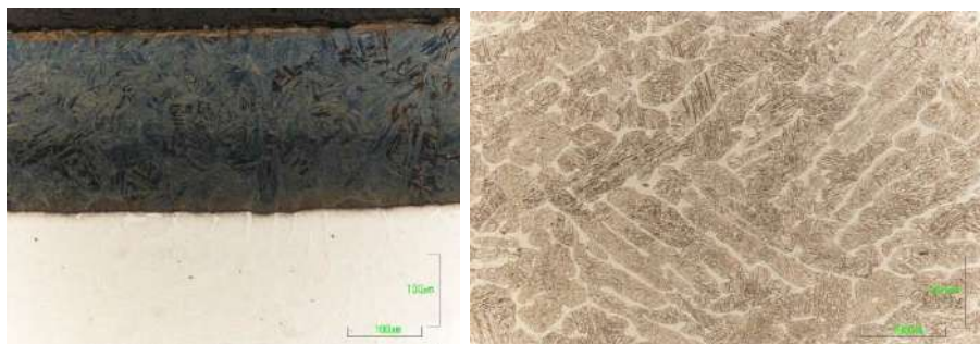
Рисунок 3. Характерный вид микроструктуры азотированного слоя
