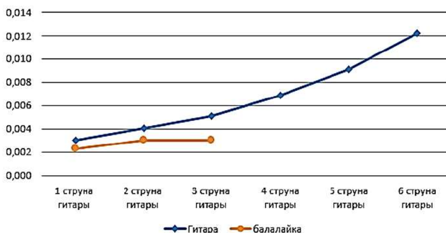
Рисунок 10. Период колебаний струн гитары и балалайки
