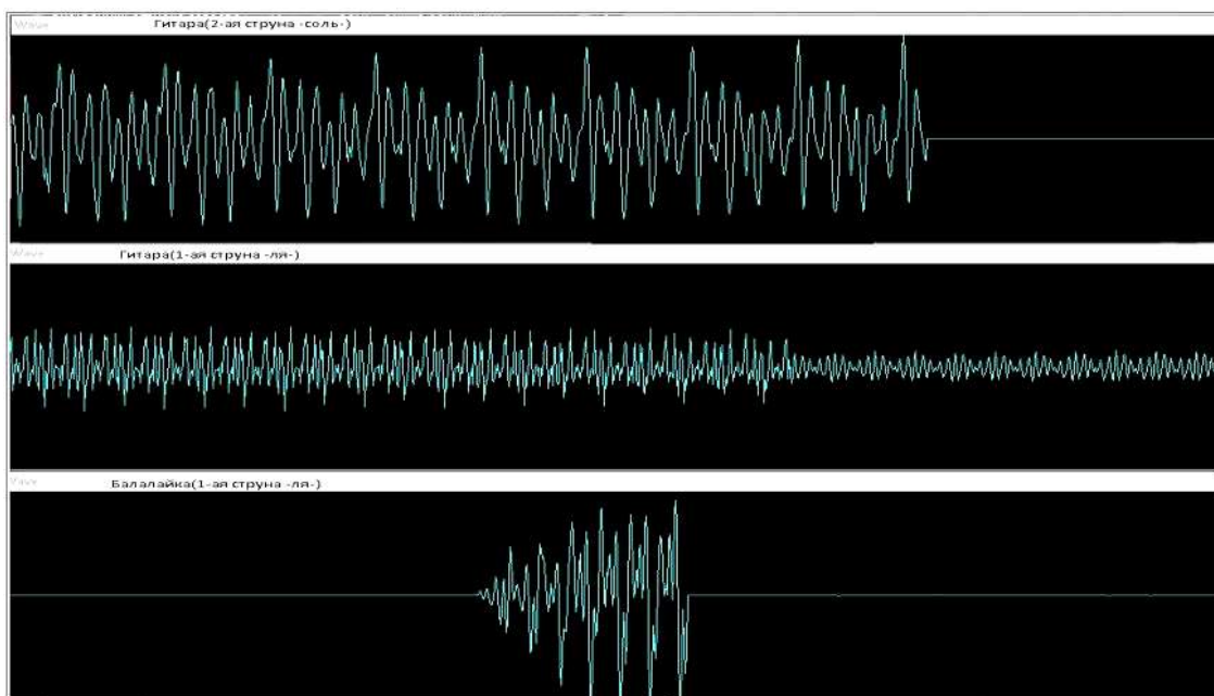
Рисунок 8. Осциллограммы колебаний 1 и 2 струн гитары и балалайки
