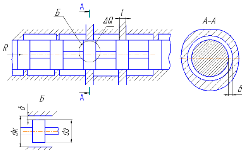
Рисунок 2. Золотник в корпусе распределителя
