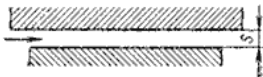
Рисунок 2. Принципиальная схема действия концентричной щели
